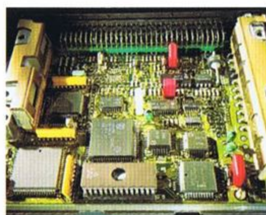
Präzises Motormanagement durch die Digitale Motor Elektronik.
