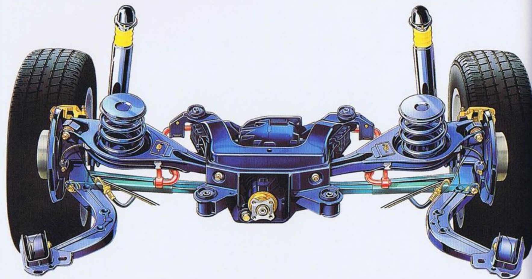
Bietet enorme Fahrstabilität und Komfort: die Zentrallenker-Hinterachse im BMW M3.
